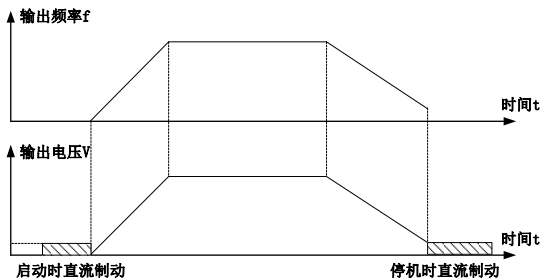
图 6-5-2 直流制动示意图
