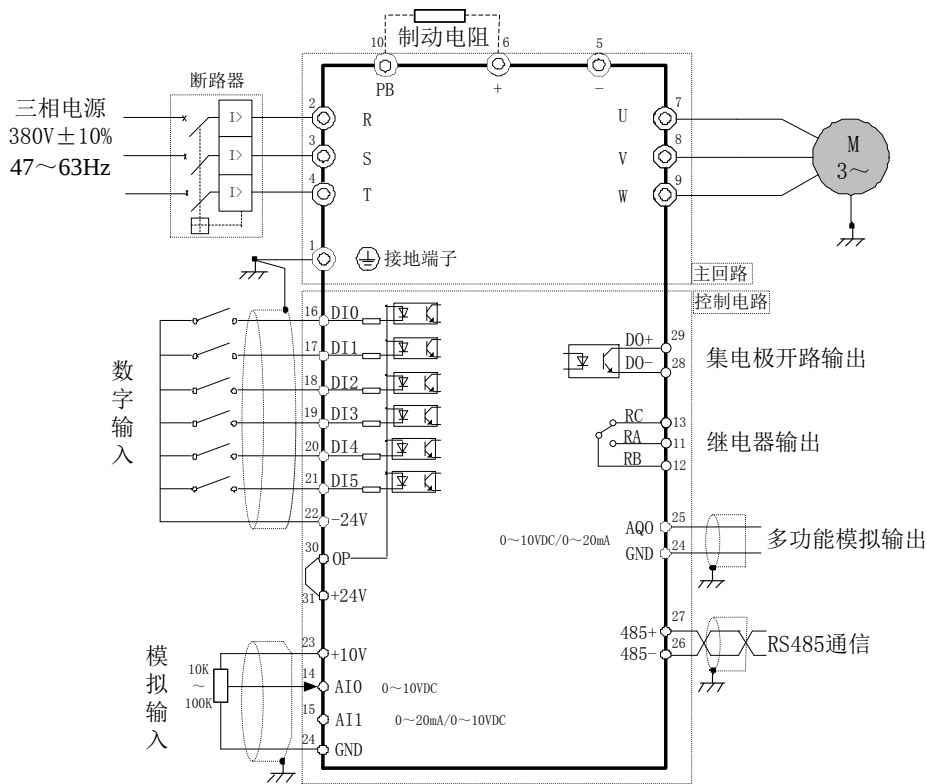
图 4-3-1 VIT_N/S 系列标准接线图
