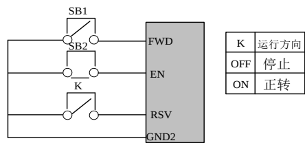
图 6-4-3 三线式运转模式 1 示意图
