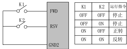
图 6-4-2 两线式运转模式 2 示意图
