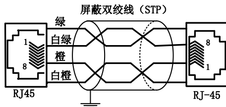
图 4-6-1 以太网接线图
