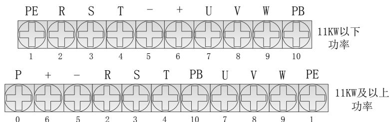
图 4-2-1 主回路端子图
