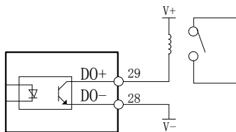
图 4-6-6 数字量输出接线
