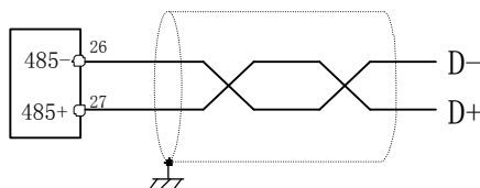
图 4-6-2 RS-485 接线方式
