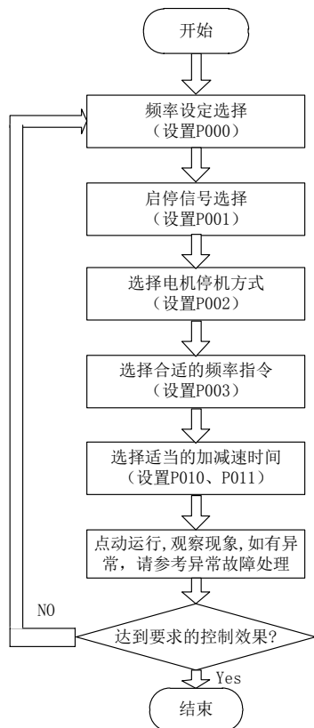
图 5-2-1 变频器快速调试流程
