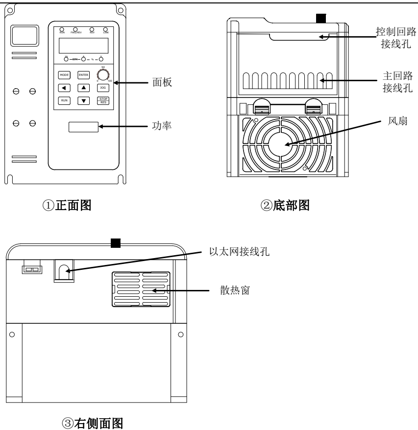
图 1-4-1 VIT_N/S 系列产品外部结构特征
