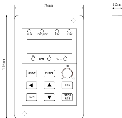
图 3-3-1 VIT_N/S 系列产品操作面板外形尺寸(单位: mm)
