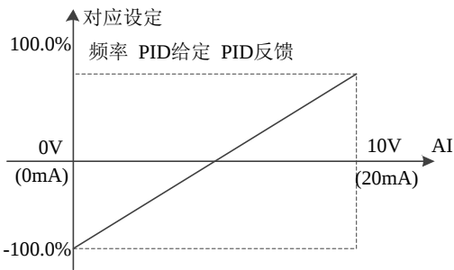
图 6-11-1 模拟给定与设定量的对应关系
