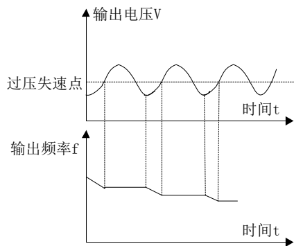
图 6-3-1 过压失速功能
