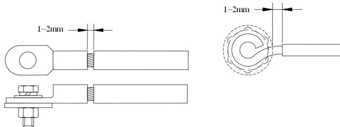
图 4-4-1 多芯线与单芯线压线方式
