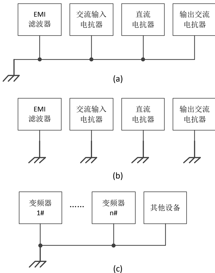
图 4-7-1 变频器附件接地方法
