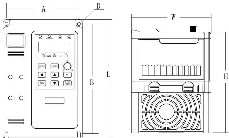
图 1-4-2 VIT_N/S 系列产品机型尺寸
