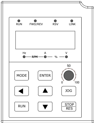
图 5-1-1 操作面板组成
