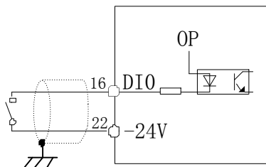
图 4-6-5 数字量输入接线
