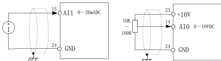
图 4-6-3 模拟量输入接线
