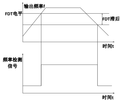
图 6-9-2 FDT 电平示意图
