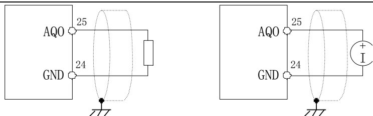
图 4-6-4 模拟量输出接线
