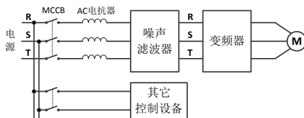
图 4-5-1 输入侧噪声滤波器接线方式
