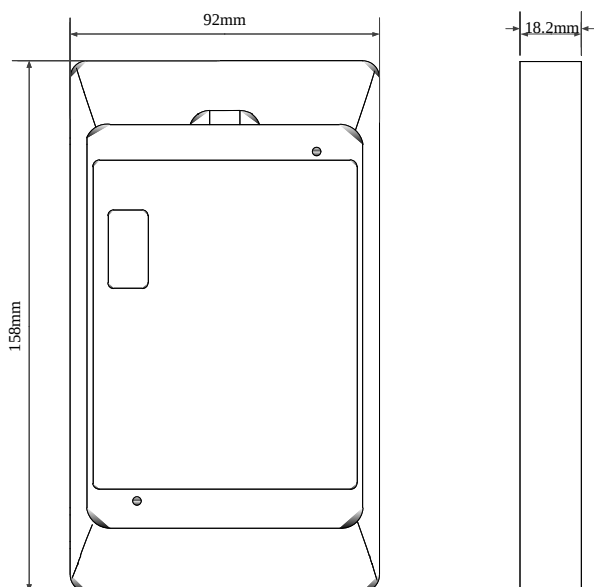
图 3-3-2 VIT_N/S 系列产品操作面板外置安装板尺寸
