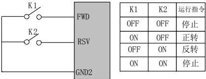
图 6-4-1 两线式运转模式 1 示意图
