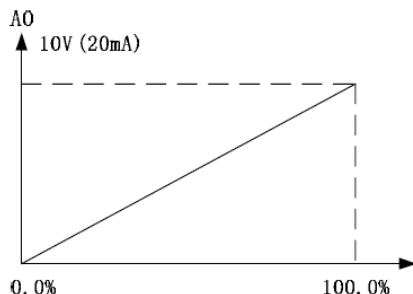
图 6-4-5 给定量与模拟量输出对应关系
