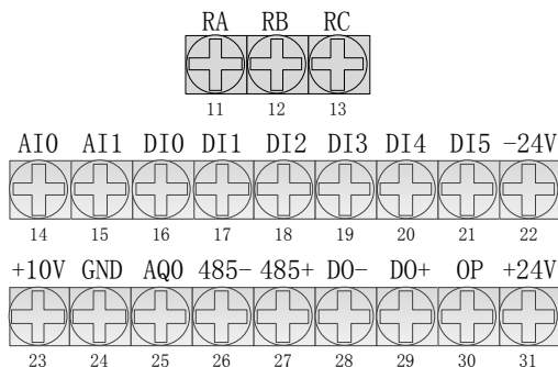
图 4-2-2 控制回路端子示意图
