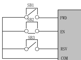
图 6-4-4 三线式运转模式 2 示意图
