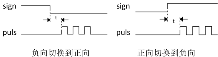
图 5-1-2 脉冲方向图
