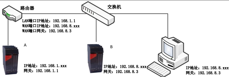
图 5-3-1 跨网段通信
