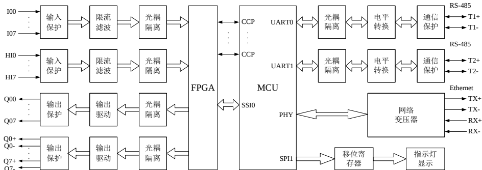
图 2-1 PEC6800 原理框图
