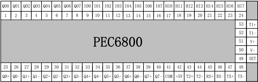
图 4-2-2 PEC6800 原理图
