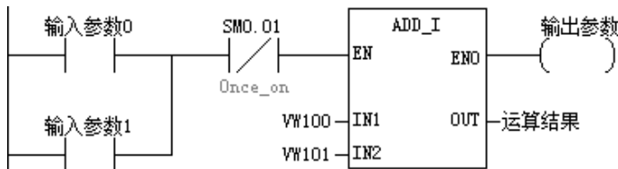
图 5-2-25 梯形图编程语言
