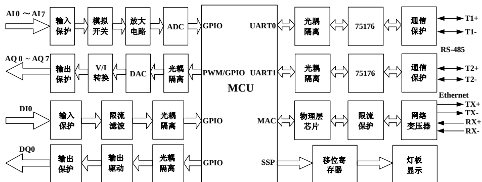
图 2-1-1 PEC5000 原理框图
