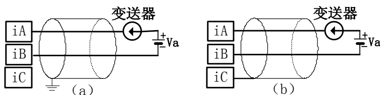
图 4-2-12 旧版 PEC5000 的电流型无源输入接线方法
