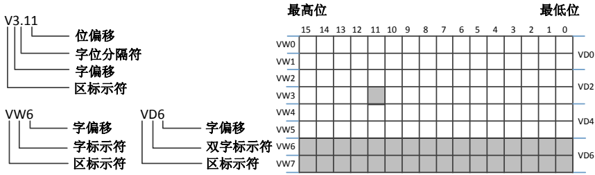
图5-2-1变量寻址示意图
