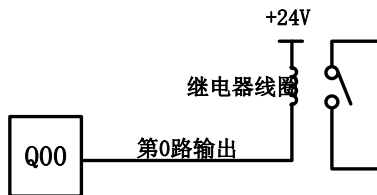
图 4-2-18 数字量输出接线方法
