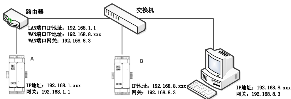
图 5-3-1 跨网段通信
