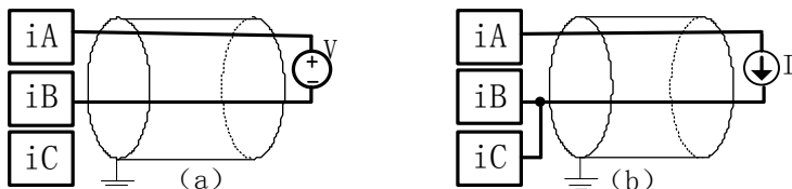
图 4-2-13 新版 PEC5000 的电压型和电流型有源输入接线方法
