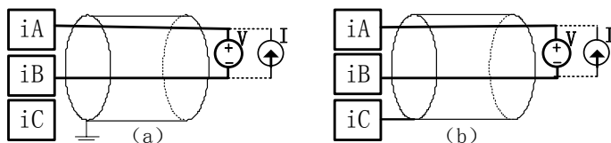
图 4-2-11 旧版 PEC5000 的电压型有源输入接线方法
