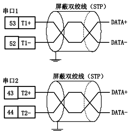
图 4-2-7 串口接线方法
