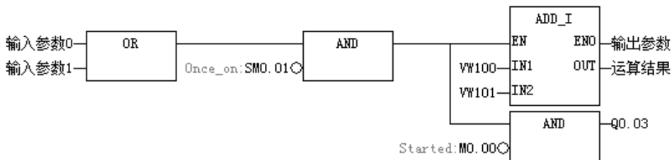
图 5-2-9 功能块编程语言
