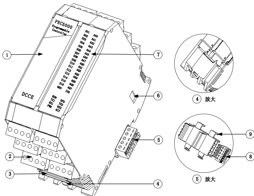
图 4-1-1 整体外观
