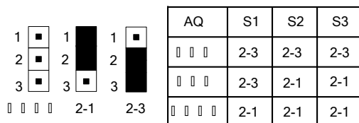
图 4-2-15AQ 输出选择内部跳线
