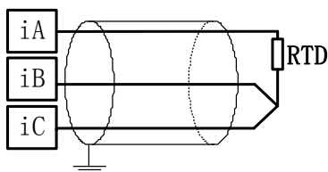
图 4-2-9 热电阻输入接线方法
