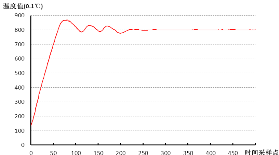
图 5-2-3 P_PID 有过冲自整定控温曲线图
