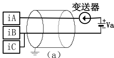
图 4-2-14 新版 PEC5000 的电流型无源输入接线方法
