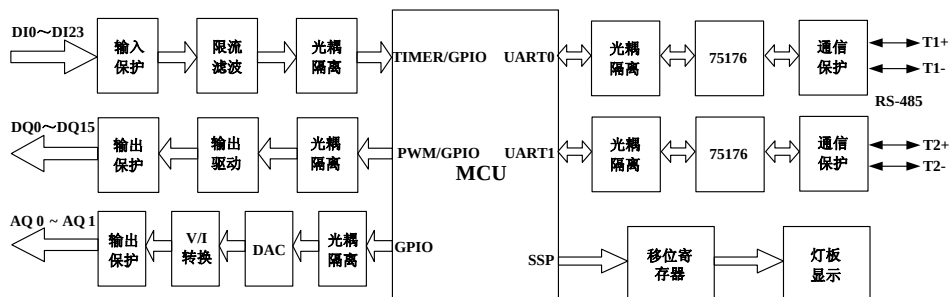
图 2-1-1 DIO3000 原理框图
