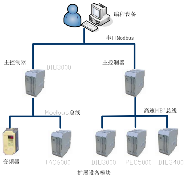
图 5-4-1 分布式控制系统
