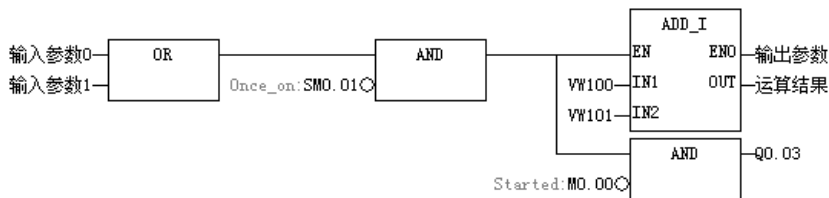
图 5-2-9 功能块编程语言
