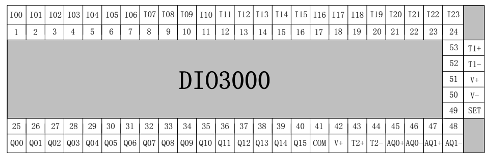
图 4-2-2 DIO3000 原理图
