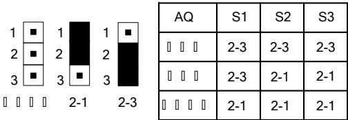
图 4-2-10 AQ 输出选择内部跳线
