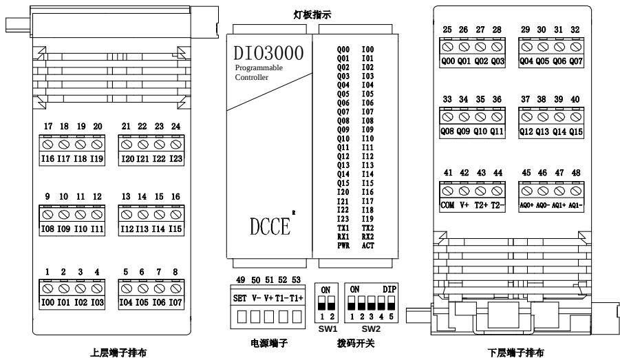
图 4-2-1 端子位置排布
