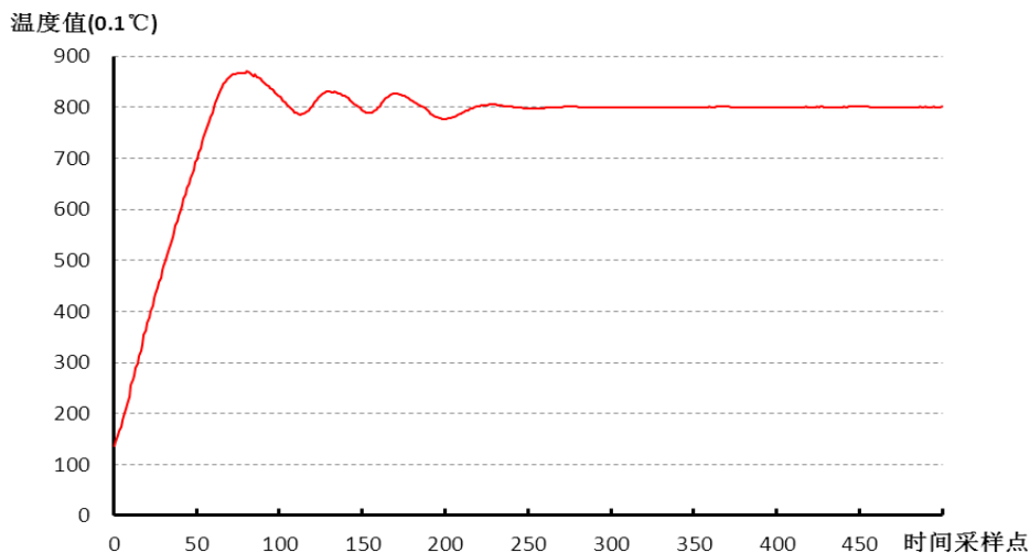
图 5-2-3 P_PID 有过冲自整定控温曲线图
