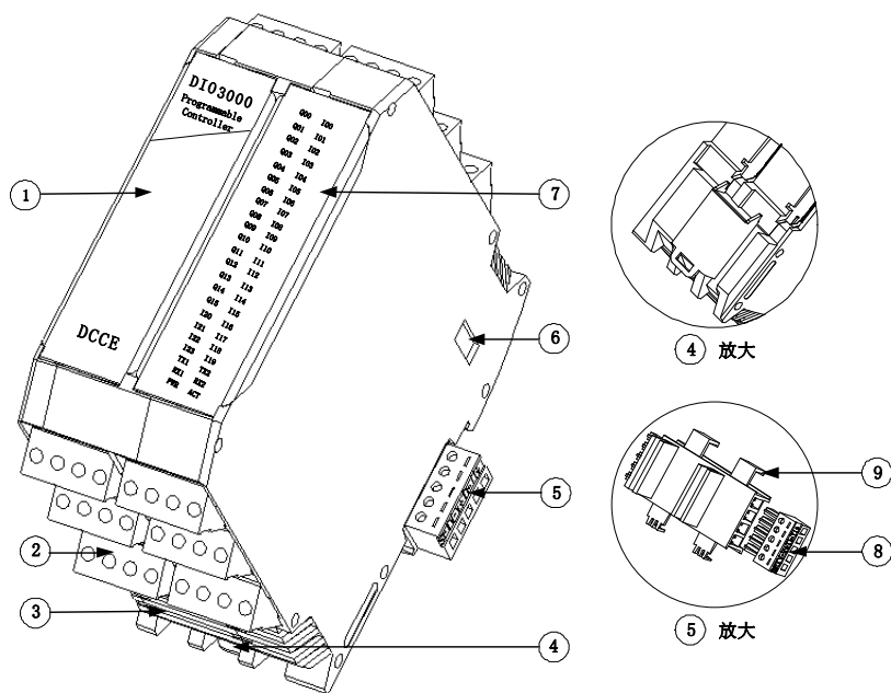
图 4-1-1 整体外观
