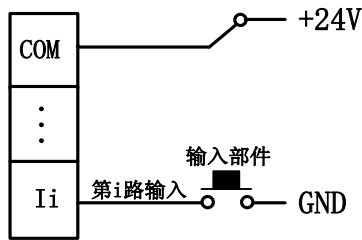
图 4-2-8 数字量输入接线方法
