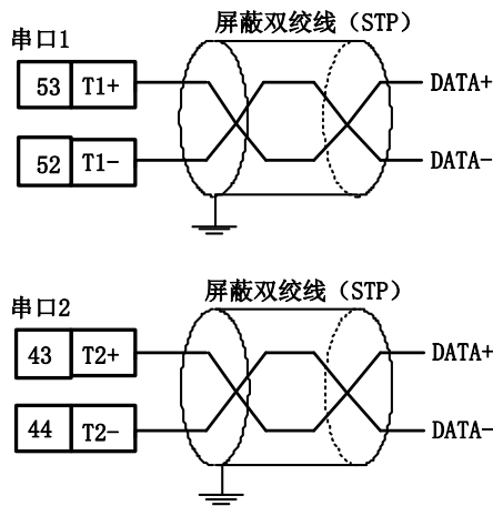
图 4-2-7 串口接线方法
