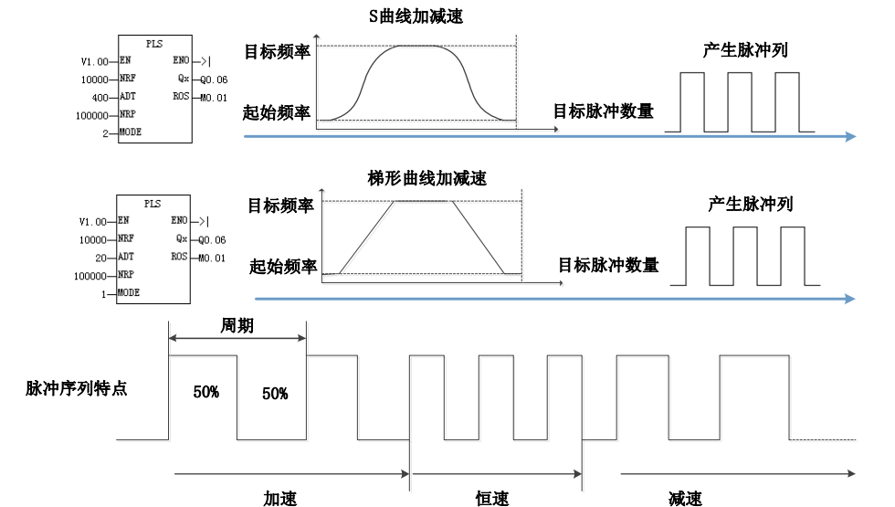
图 5-2-6 高速输出方式
