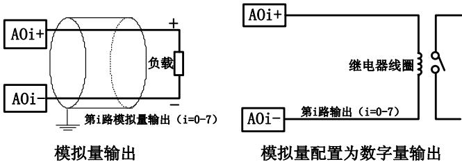
图 4-2-11 模拟量输出接线方法
