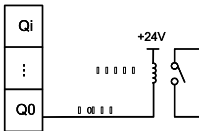
图 4-2-9 数字量输出接线方法
