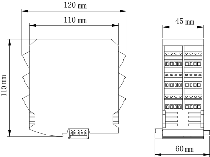
图 4-1-2 外形尺寸
